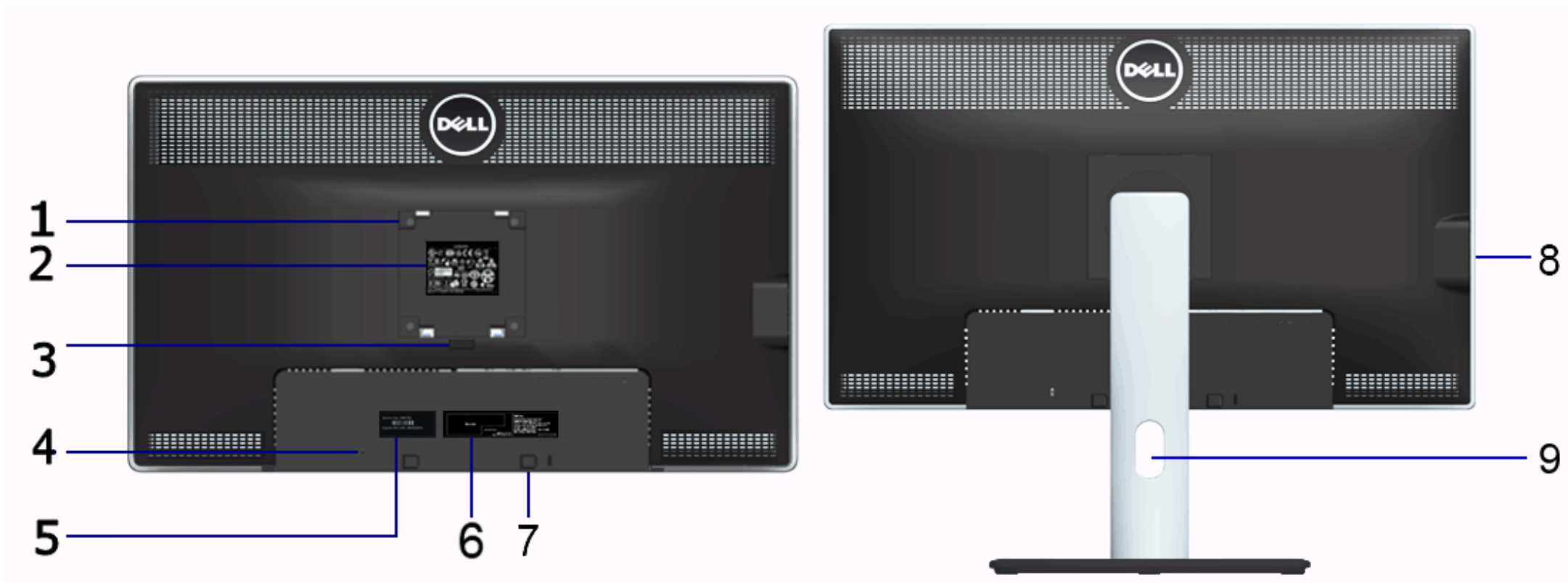
背視圖
